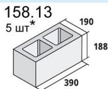
Камень стеновой
