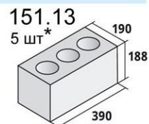
Камень стеновой
