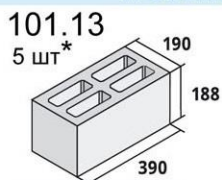
Камень стеновой
