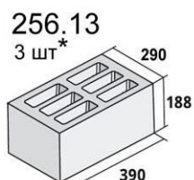
Блок стеновой
