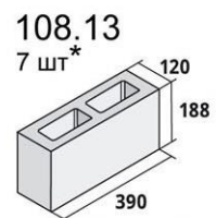
Полублок стеновой
