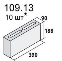
Полублок стеновой
