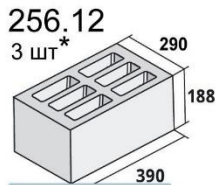
Блок стеновой
