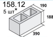
Камень стеновой
