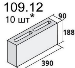
Полублок стеновой
