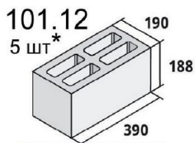
Камень стеновой
