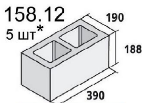
Камень стеновой
