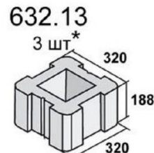
Элемент столба
