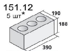
Камень стеновой
