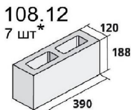
Полублок стеновой
