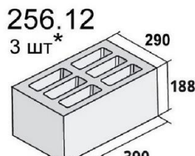
Блок стеновой
