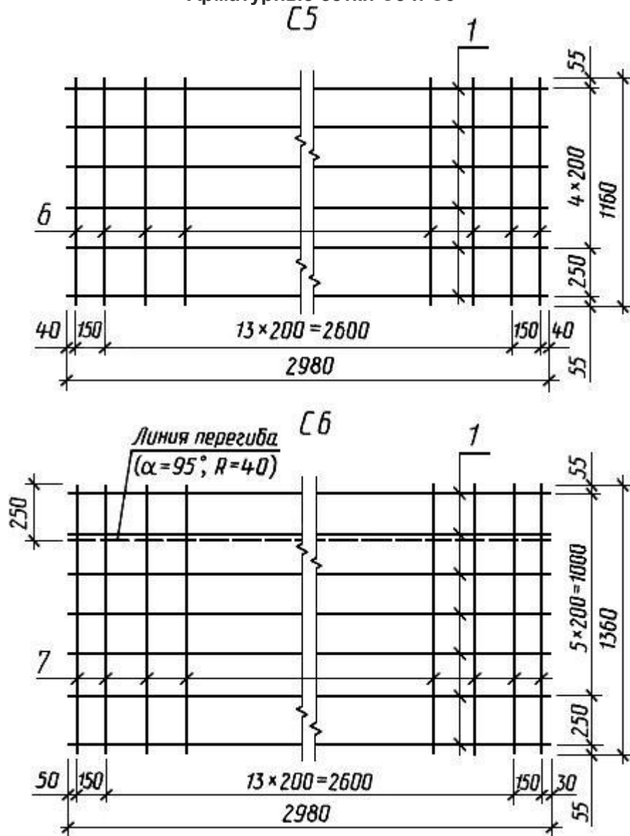
Арматурные сетки С5 и С6
