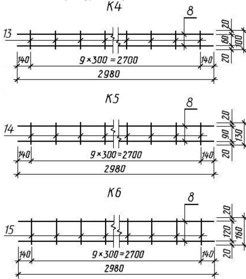
Арматурные каркасы К4, К5 и К6
