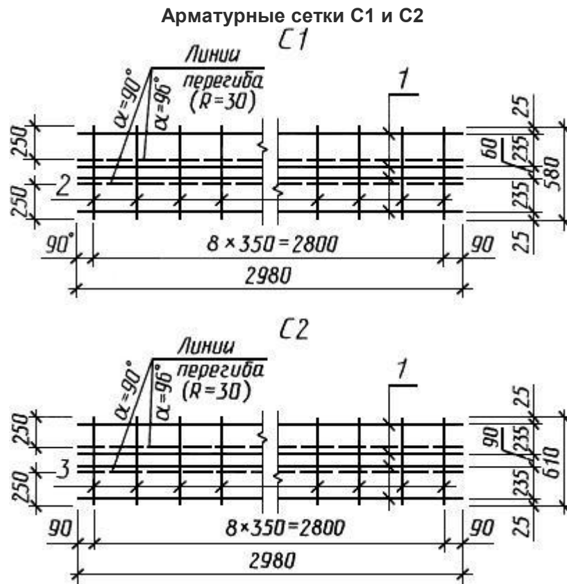
Черт.29. Арматурные сетки С1 и С2
