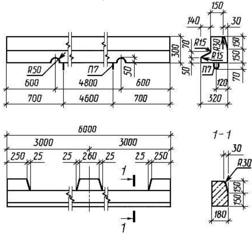
Камни марки БУП600.30.32-A-IV
