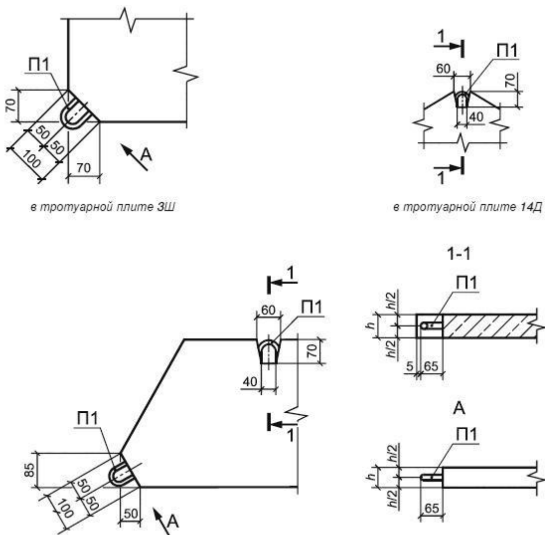
Рисунок Б.1 - Детали установки петель П1
