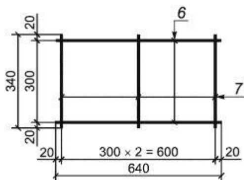
Рисунок Б.12 - Арматурная сетка С10
