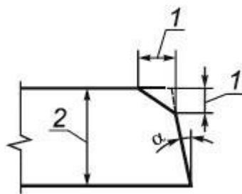
Рисунок 1 - Пример фаски и бокового скоса (уклона)
