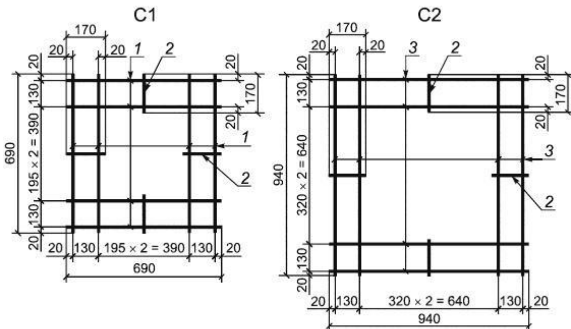
Рисунок Б.8 - Арматурные сетки С1, С2
