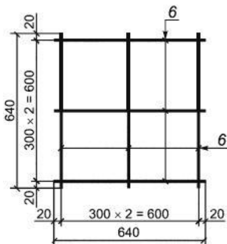
Рисунок Б.10 - Арматурная сетка С6
